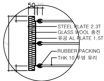
A 부분 상세 SCALE : 1 / NONE
