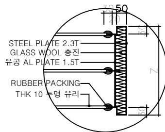
B 부분 상세 SCALE : 1 / NONE
