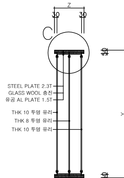
단면상세도 (SCALE 1/20)
