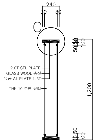
단면상세도 (SCALE 1/20)
