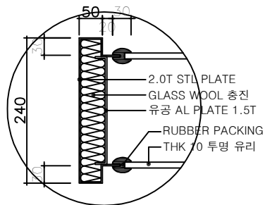
A 부분 상세 SCALE : 1 / NONE
