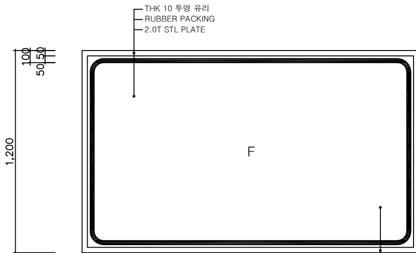
방음시창 입면도 (SCALE 1/20)
