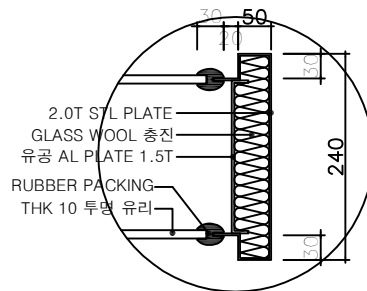
B 부분 상세 SCALE : 1 / NONE
