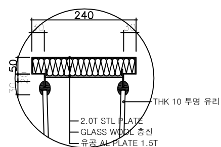
C 부분 상세 SCALE : 1 / NONE
