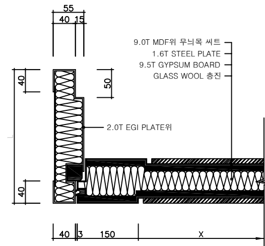
JAMB SECTION (SCALE 1/5)
