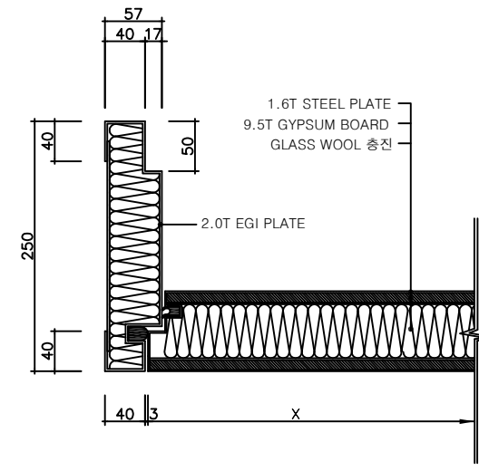
JAMB SECTION (SCALE 1/5)
