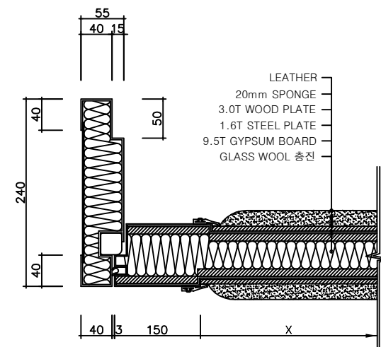
JAMB SECTION (SCALE 1/5)
