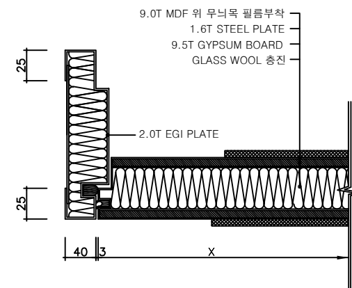
JAMB SECTION (SCALE 1/5)
